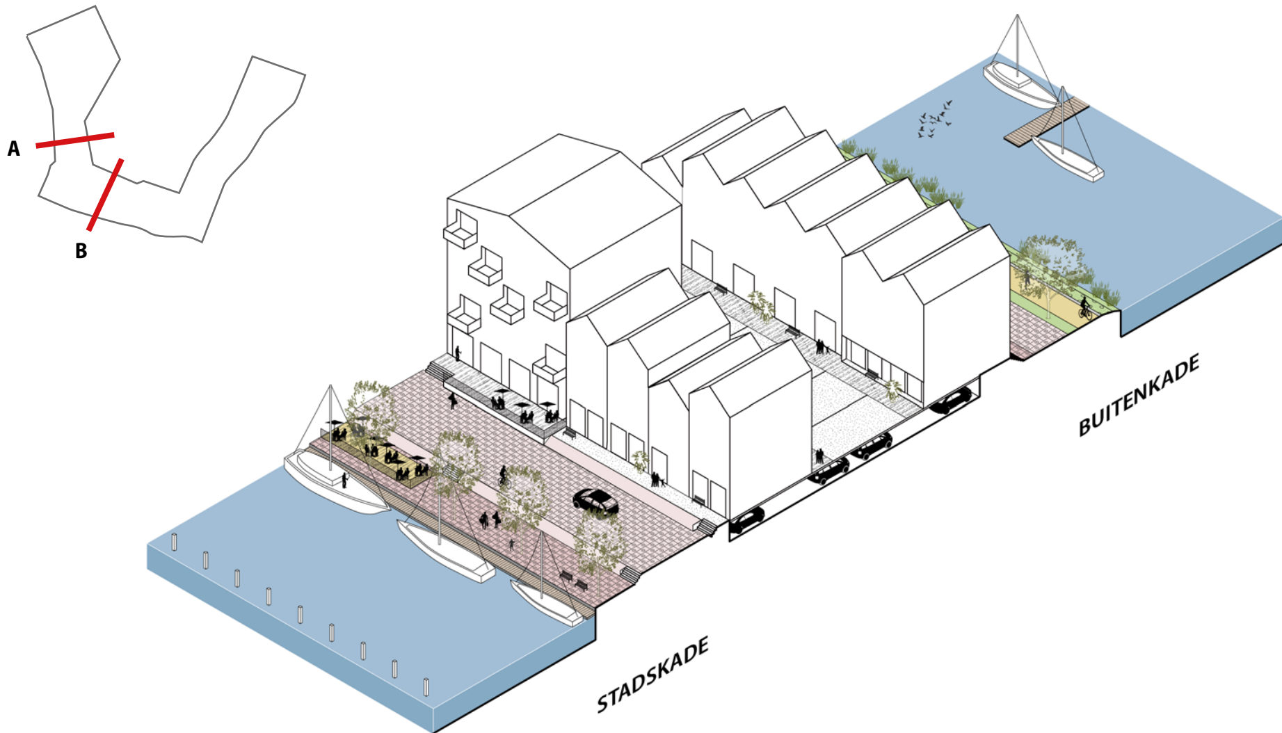
DOORSNEDE A
